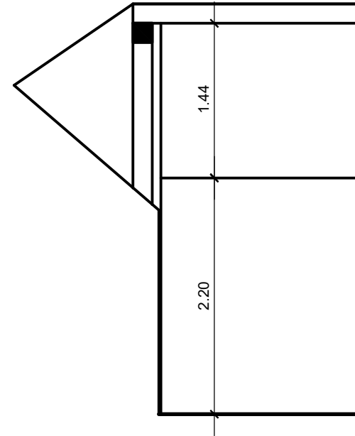
Schnitt A-A
