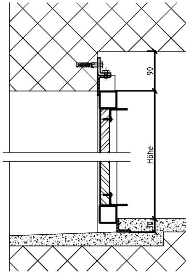
Vertikalschnitt
