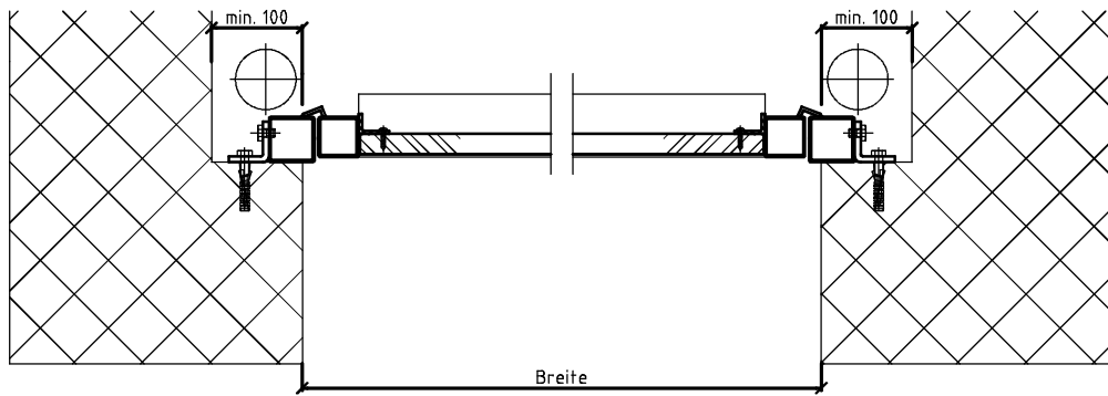
Horizontalschnitt
