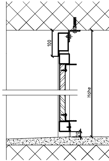
Vertikalschnitt
