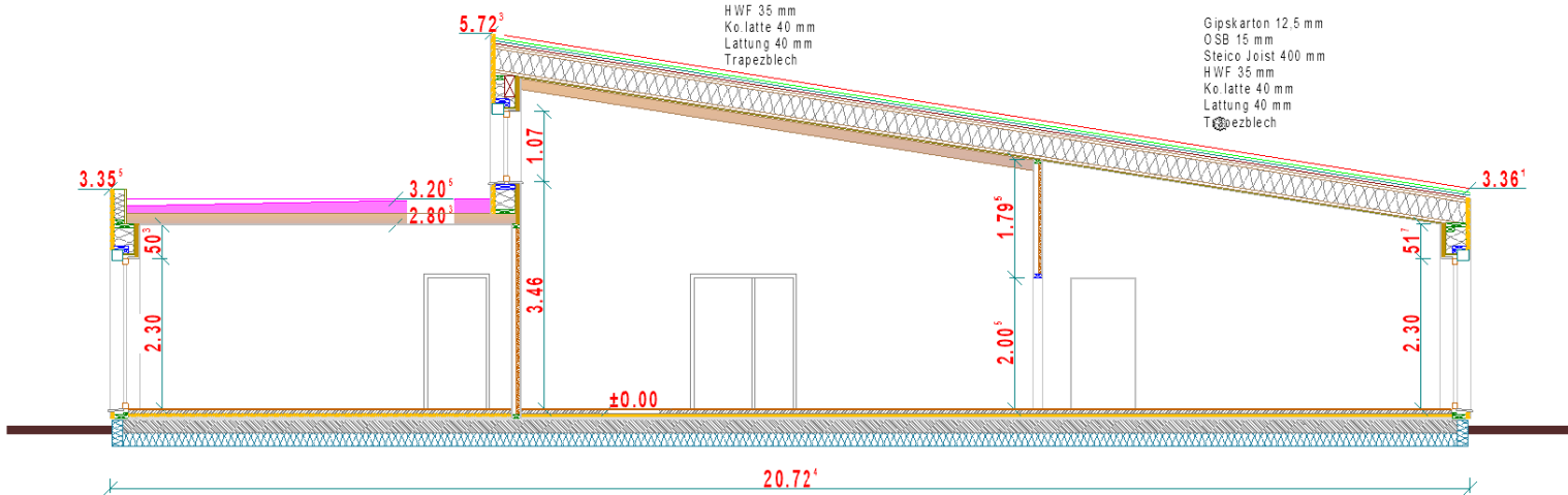
Schnitt, Ansicht
