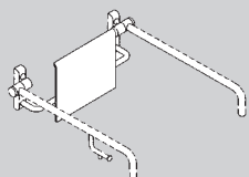
Montage in Verbindung mit Stützklappgriffen Mounting accessories (for use with 2 cantilever rails)
