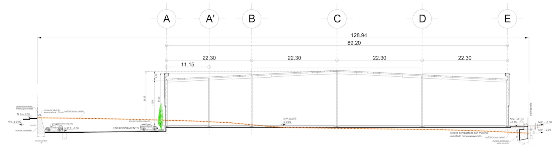
CORTE F-F'
