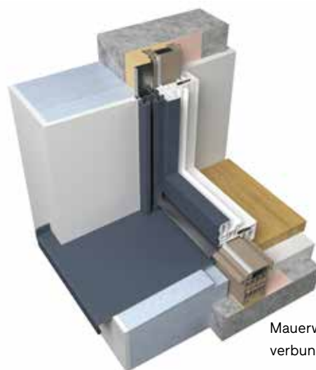
monolithisches Mauerwerk
