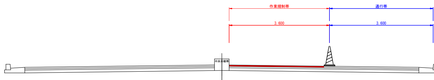
【標準断面図】
