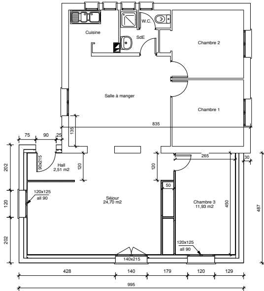
Echelle : 1 / 50 (2 cm = 1 m)
