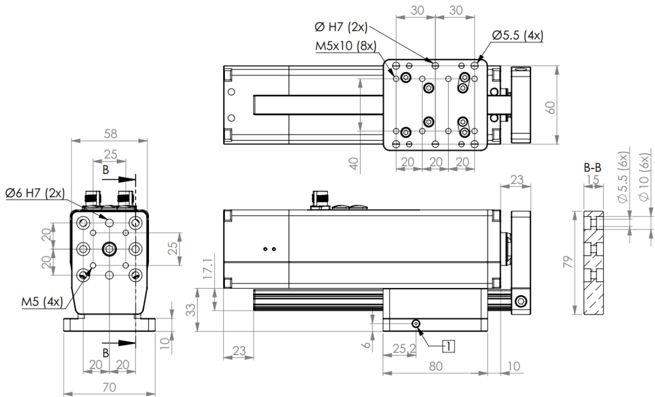
FIGURE 5: DIMENSIONS CTC-___-___-___-F
