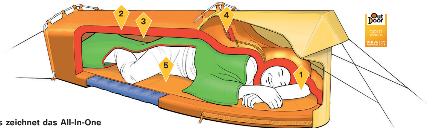
Schnittbild Polarmond® All-In-One Biwak
