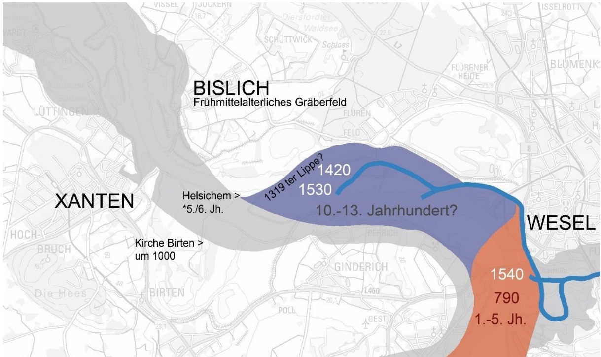
Die mittelalterliche Aue zwischen Bislich und Spellen mit historischen Verläufen und Mündungen der Lippe. Entwurf: Peter Bruns.
