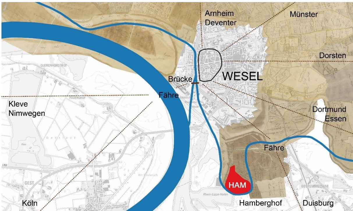
Lage des Hams in der Lippeaue südlich von Wesel im Kataster Kleve von 1735 mit Rekonstruktionsvorschlag des Lippelaufes von 1317. Entwurf: Peter Bruns
