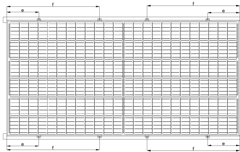
Figure 5: 394\text{mm} < e < 444\text{mm} 、 914\text{mm} < f < 964\text{mm}
