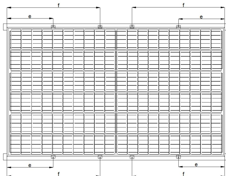
Figure 5: 212\text{mm} < e < 262\text{mm} 、 732\text{mm} < f < 782\text{mm}
