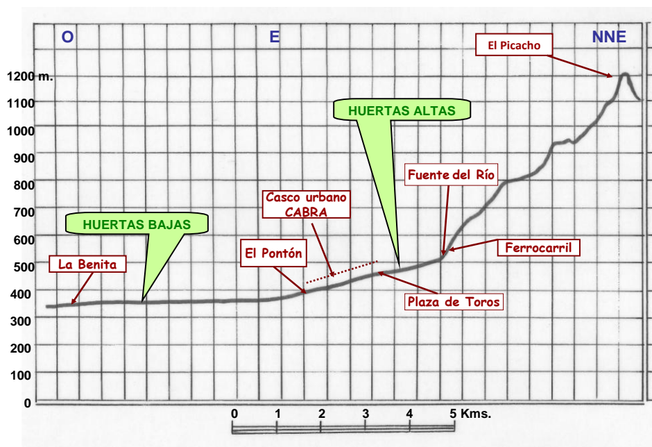
Fig. 1.-Perfil Topográfico desde el límite occidental del municipio de Cabra hasta El Picacho
