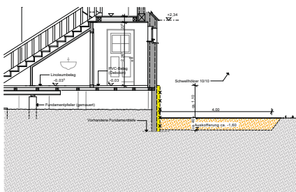
Schritt 2: Vormauerschale abnehmen (zur Wiederverwendung)
