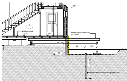
Schritt 3: Verbau (Trägerbohlenwand) abteufen und Abfangjoche für aufgehendes Mauerwerk herstellen (je 2 x HEB 200)
