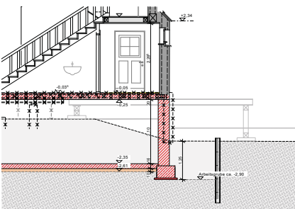
Schritt 10: Holzbalkendecke abschnittsweise abbrechen neue Betondecke C20/25 einbauen
