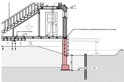
Schritt 8: Joche umsetzen und Keller abschnittsweise auskoffern
