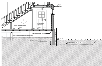
Schritt 1: Arbeitsebene herstellen (auskoffern)
