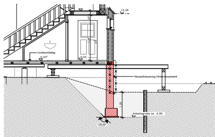
Schritt 7: Mauerstufen abschnittsweise entfernen und ausmauern bzw. ausbetonieren
