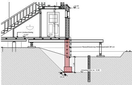
Schritt 6: Hintermauerwerk 36,5 cm NF im Pilgerschrittverfahren abschnittsweise herstellen (incl. Verzahnung)
