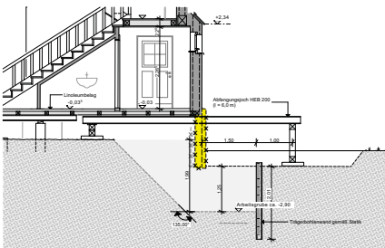
Schritt 4: Arbeitsgrube für Unterfangung herstellen (max. 1,20m breit / Böschungswinkel innen max. 45°) und Hintermauerwerk sukzessive abbauen
