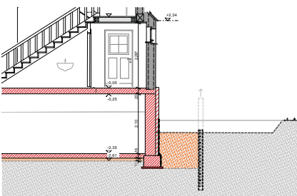
Schritt 12: Abstützungen ausbauen, Verbau entfernen und Baugrube füllen
