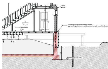
Schritt 9: neue Betonschle C20/25 (incl. Perimeterdämmung Foamglas) abschnittsweise einbauen
