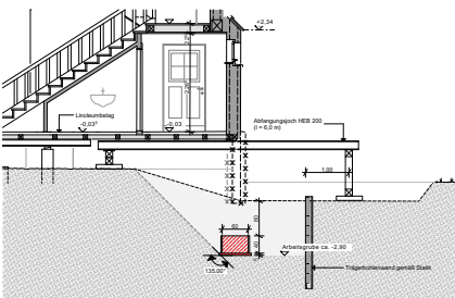
Schritt 5: Stahlbeton-Streifenfundament C 20/25 im Pilgerschrittverfahren abschnittsweise herstellen (incl. Sauberkeitschicht und Schalung)
