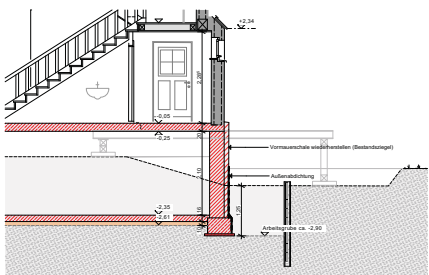
Schritt 11: Vormauerschale herstellen (incl. Außenabdichtung)
