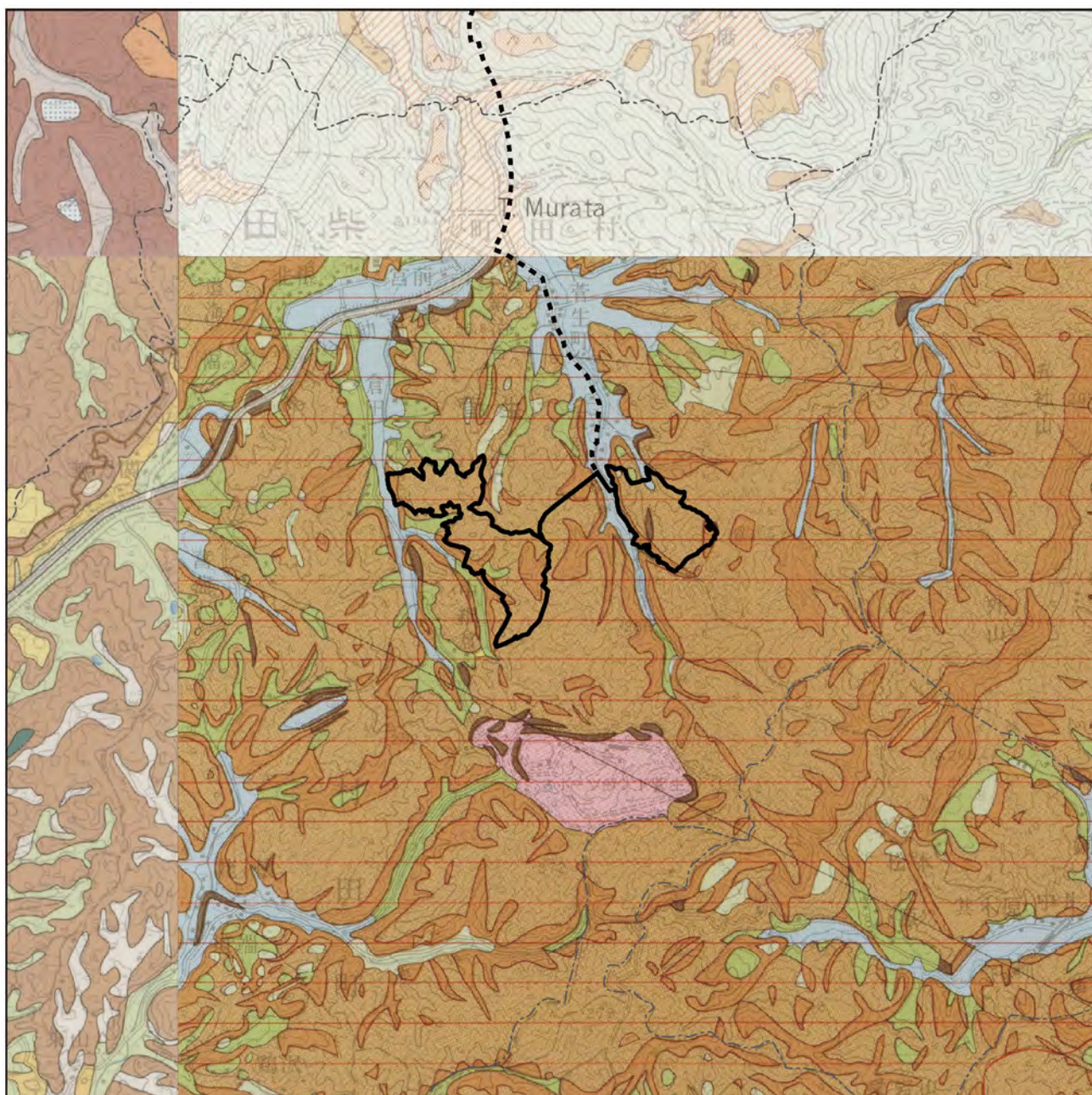
図 4.3-1 地形の状況
