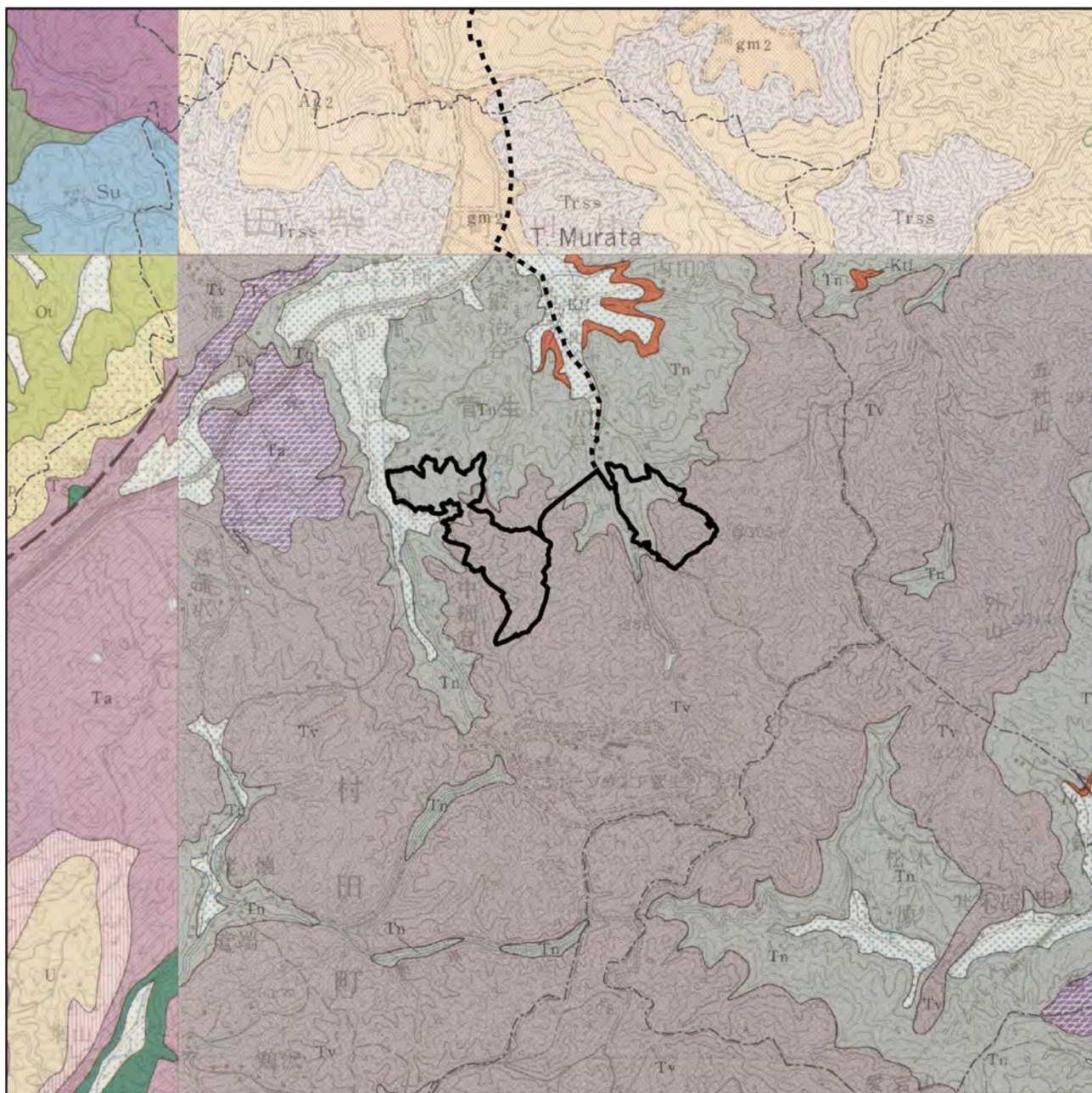
図 4.3-2 地質の状況
