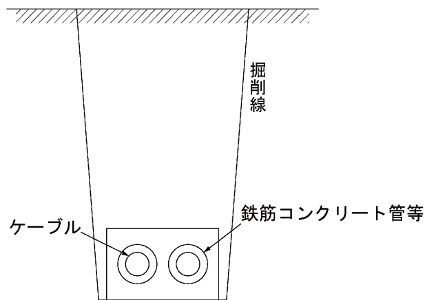
図2.2-9 管路式の自営線敷設イメージ
