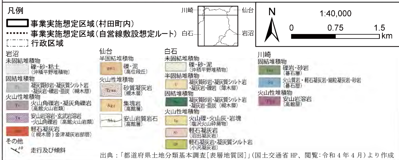
図 4.3-2 地質の状況
