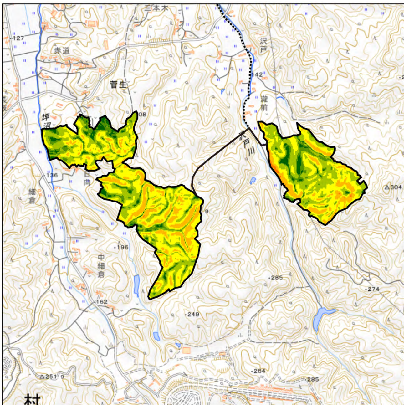
図 4.3-5 傾斜区分図
