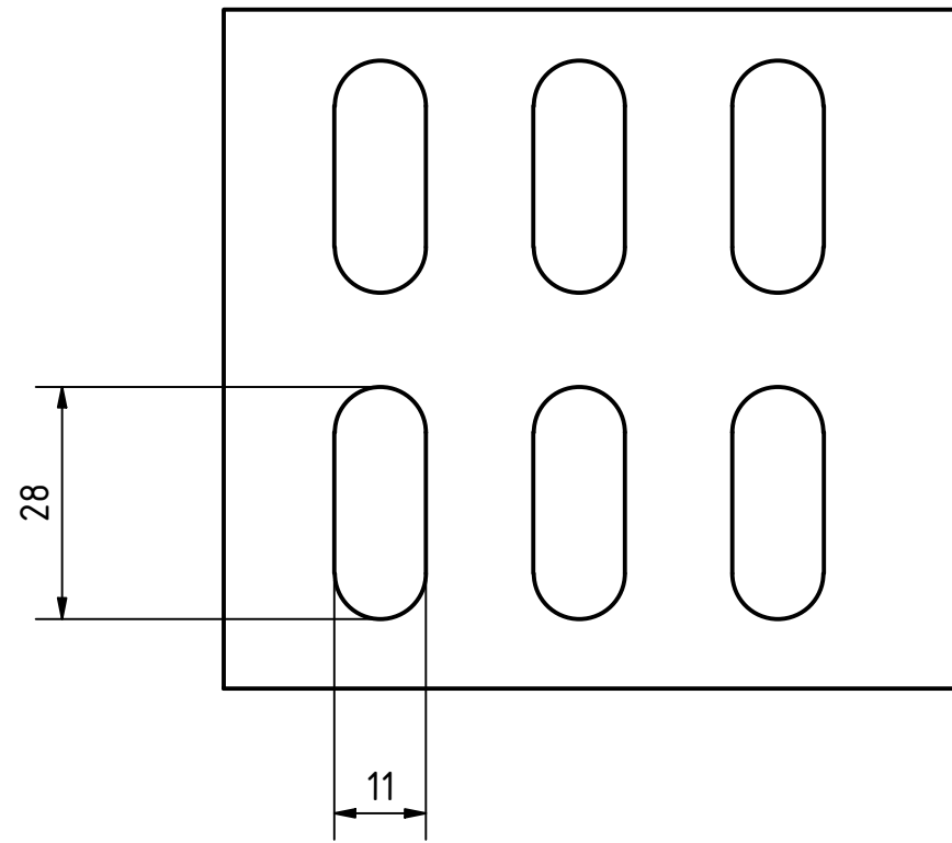
Lochbild ( 1: 1 )
