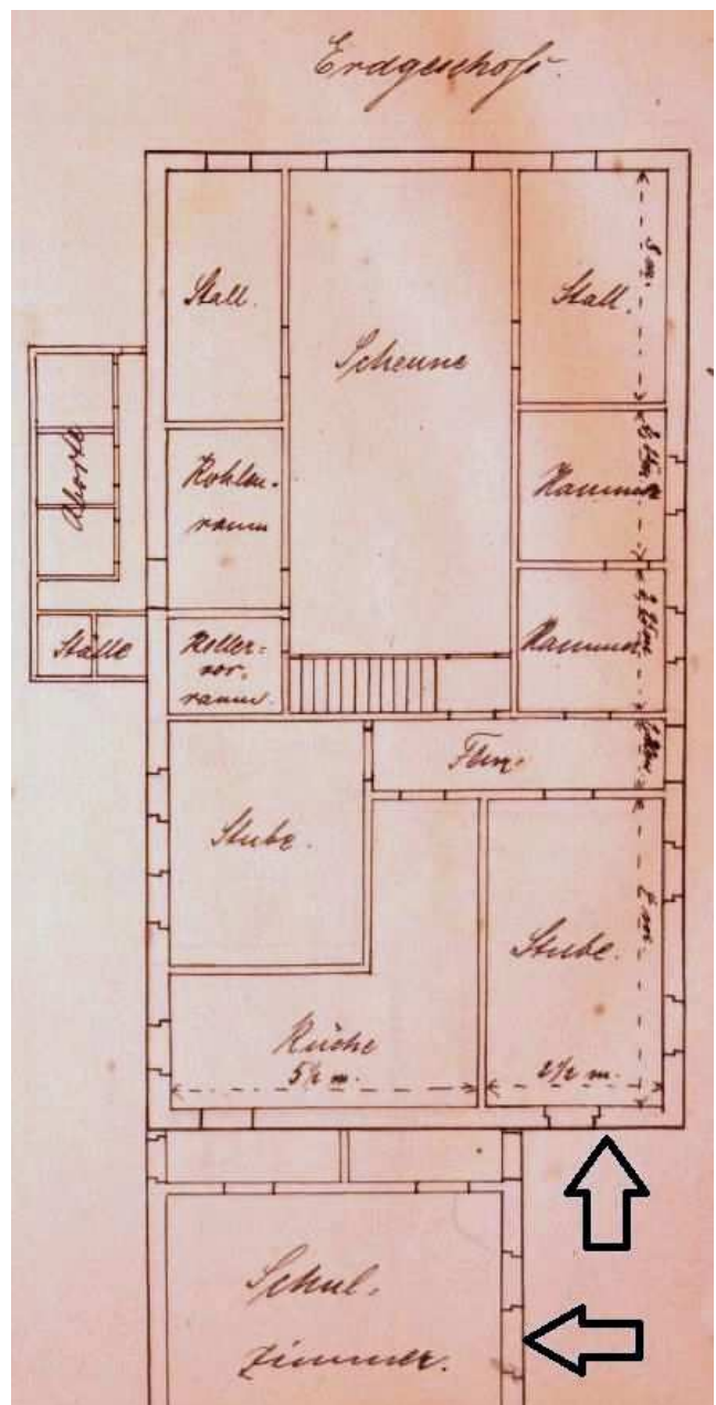
Bild 6 1 : (Ausschnitt, ergänzt) Erdgeschoss. Ein Schulzimmer wurde an der Südwand angebaut und das ehemalige Schulzimmer als Stube genutzt.
