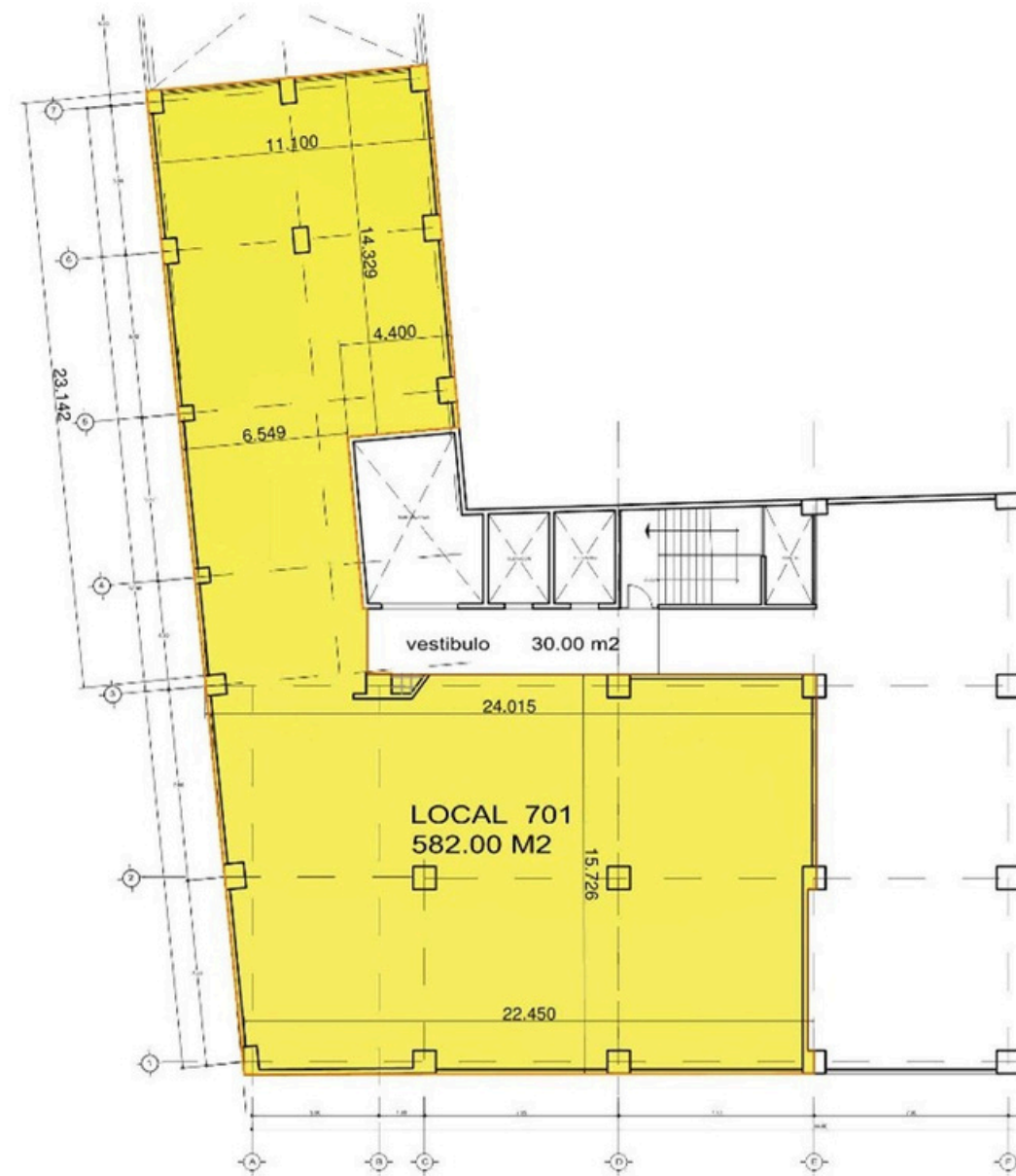
DETALLE DEL LOCAL
