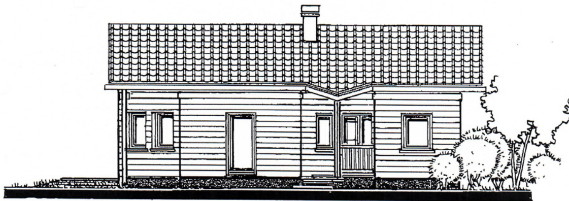
OSTANSICHT
