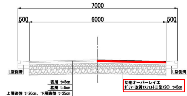
標準断面図 S=1/30(A1)、S=1/80(A3)
