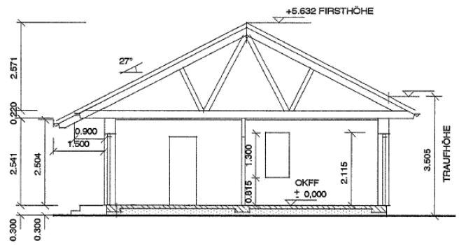
SCHNITT
