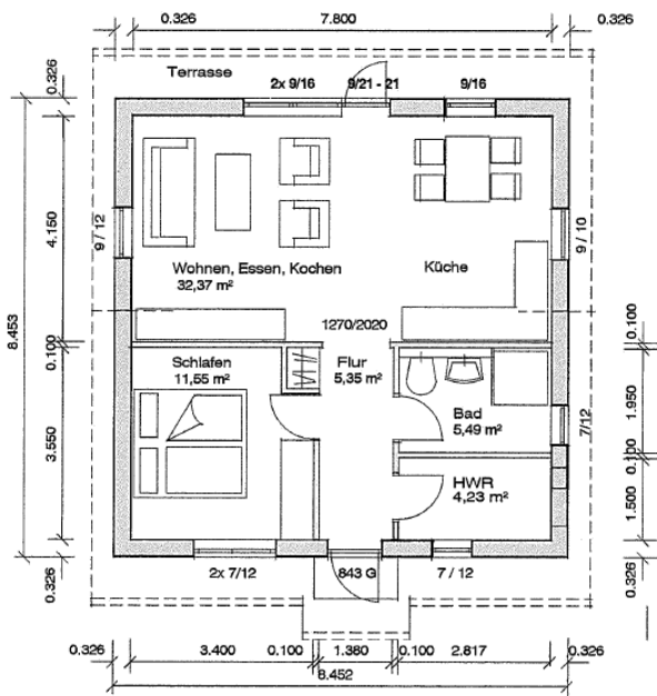
ERDGESCHOSS
