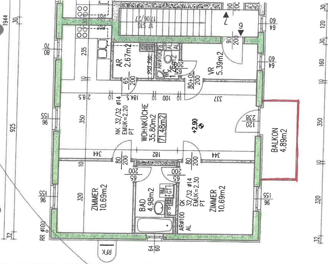
OBERGESCHOSS, M 1:100
