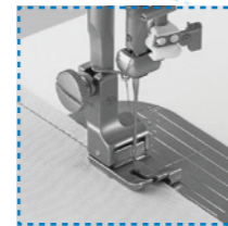
AUSGLEICHFUß
