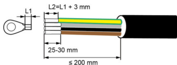
Abbildung 5-9 Vieradriges Kabel (mit Erdungskabel, jedoch ohne Neutralleiter)
