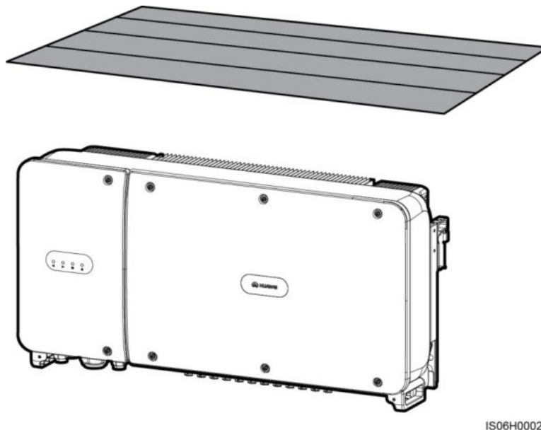
Abbildung 4-2 Vordach
