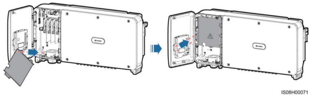
Abbildung 5-39 Montieren einer Abdeckung
