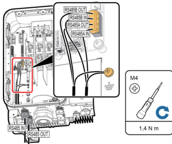
Abbildung 5-28 Anschließen der Kommunikationskabel
