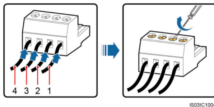
Abbildung 5-27 Anschließen von Kabeln an eine Klemmenbasis
