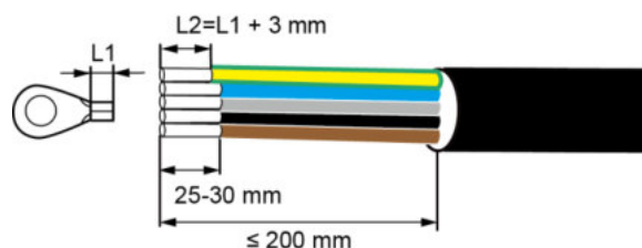
Abbildung 5-11 Fünfadriges Kabel (mit Erdungskabel und Neutralleiter)
