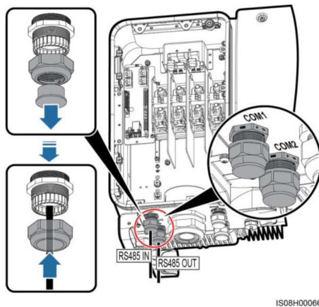
Abbildung 5-26 Verlegen eines Kabels
