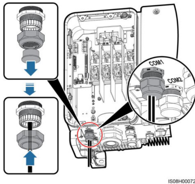
Abbildung 5-32 Verlegen eines Kabels
