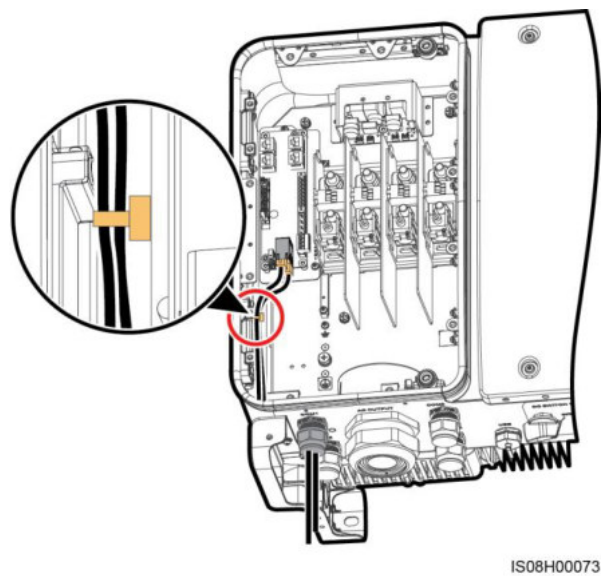
Abbildung 5-34 Bündeln der Kommunikationskabel
