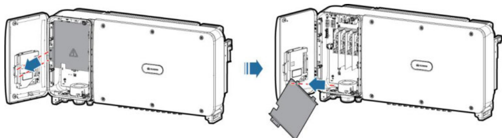
Abbildung 5-5 Entfernen einer Abdeckung
