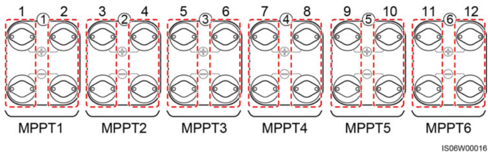
Abbildung 5-17 DC-Klemmen
