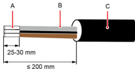
Abbildung 5-8 Dreifadriges Kabel (ohne Erdungskabel und Neutralleiter)
