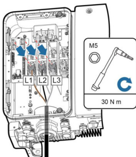
Abbildung 5-13 Dreiadriges Kabel (ohne Erdungskabel und Neutralleiter)
