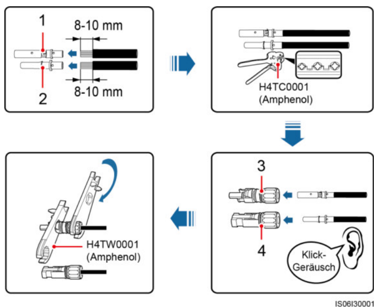
Abbildung 5-18 Vorbereiten von Plus- und Minus-Steckverbindern (mit kaltumformendem Kontakt)
