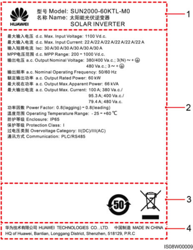
Abbildung 2-3 Typenschild
