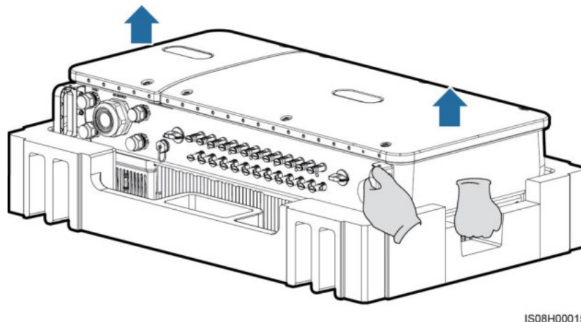
Abbildung 4-16 Herausnehmen eines SUN2000
