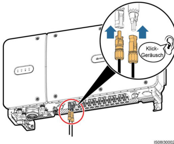
Abbildung 5-21 Anschließen der DC-Eingangsstromkabel
