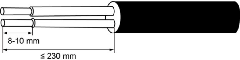
Abbildung 5-25 Abisolieren eines RS485-Kommunikationskabels
