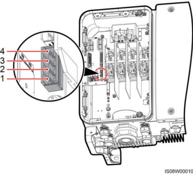
Abbildung 5-24 Klemmleiste
