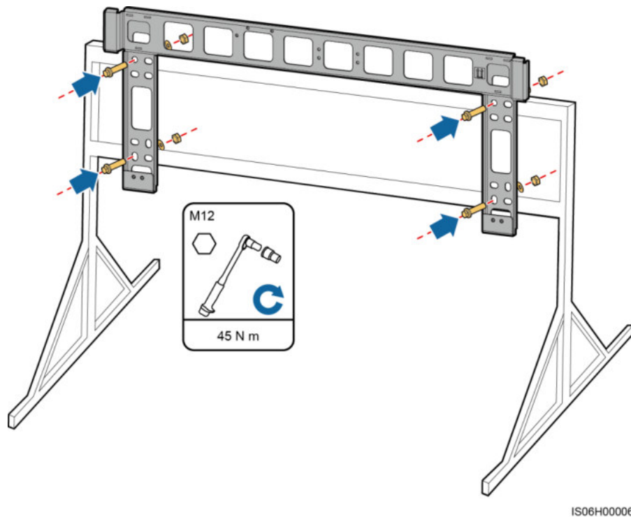
Abbildung 4-12 Befestigen einer Montagehalterung
