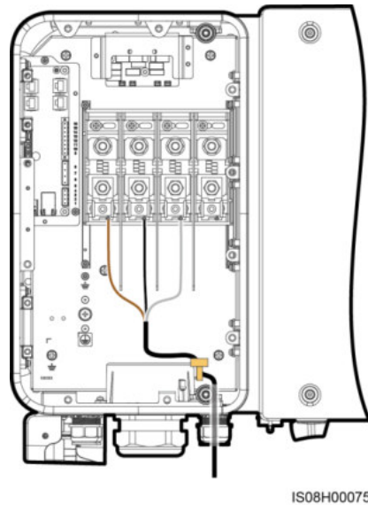
Abbildung 5-38 Binden eines Netzkabels des Solar-Trackers
