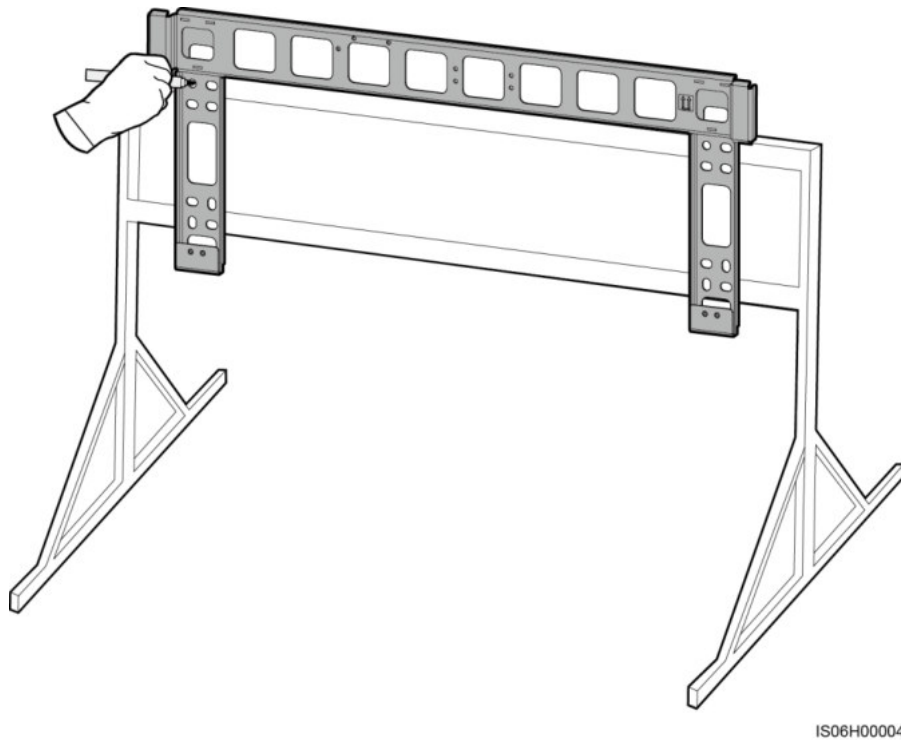
Abbildung 4-10 Ermitteln der Lochpositionen
