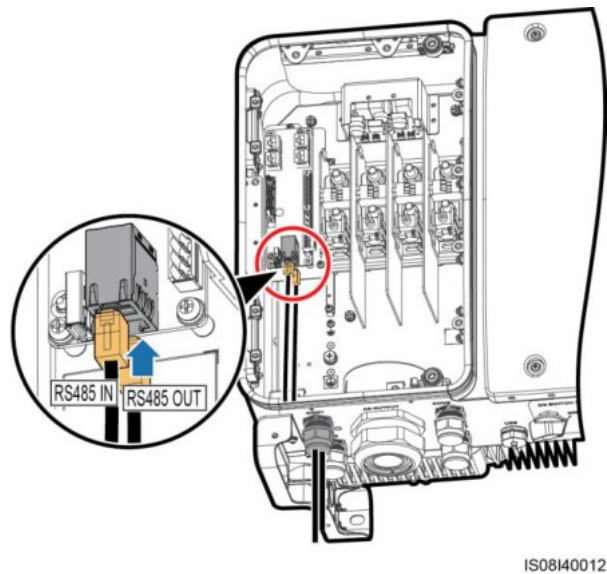
Abbildung 5-33 Anschließen der Kommunikationskabel
