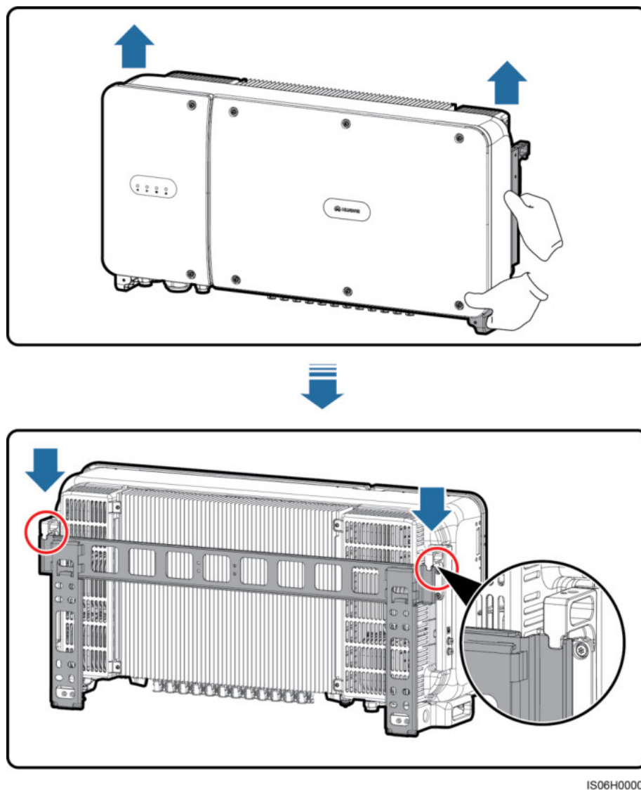
Abbildung 4-18 Montieren des SUN2000 an eine Montagehalterung
