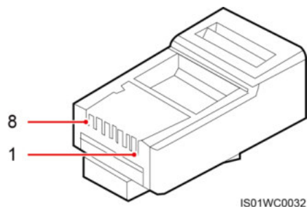
Abbildung 5-30 RJ45-Steckverbinder
