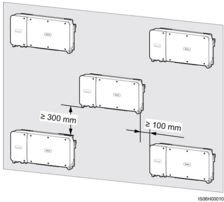
Abbildung 4-6 Dreiecks-Montagemethode (empfohlen)
