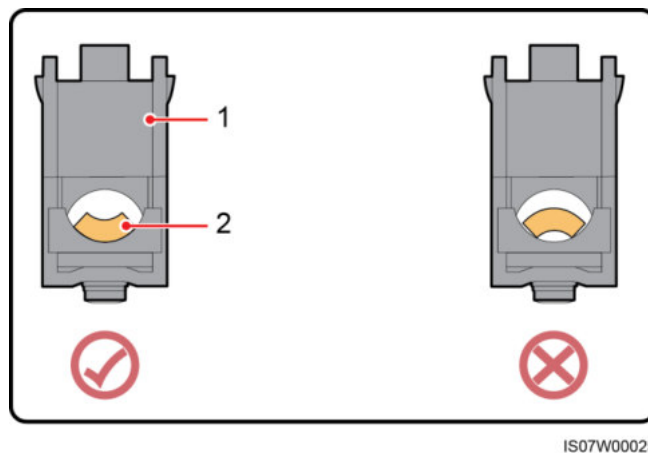
Abbildung 5-12 Montageanforderungen für das AC-Ausgangsstromkabel
