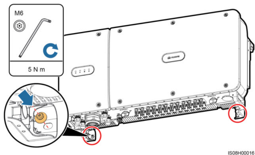
Abbildung 4-19 Anziehen der Diebstahlschutzschrauben
