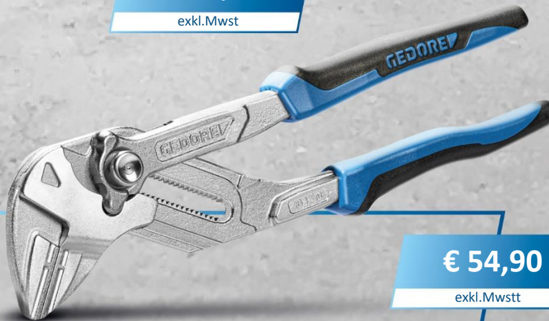
3112268 ZANGENSCHLÜSSEL 10" INKL. 4 SCHONBACKEN 5-teilig
