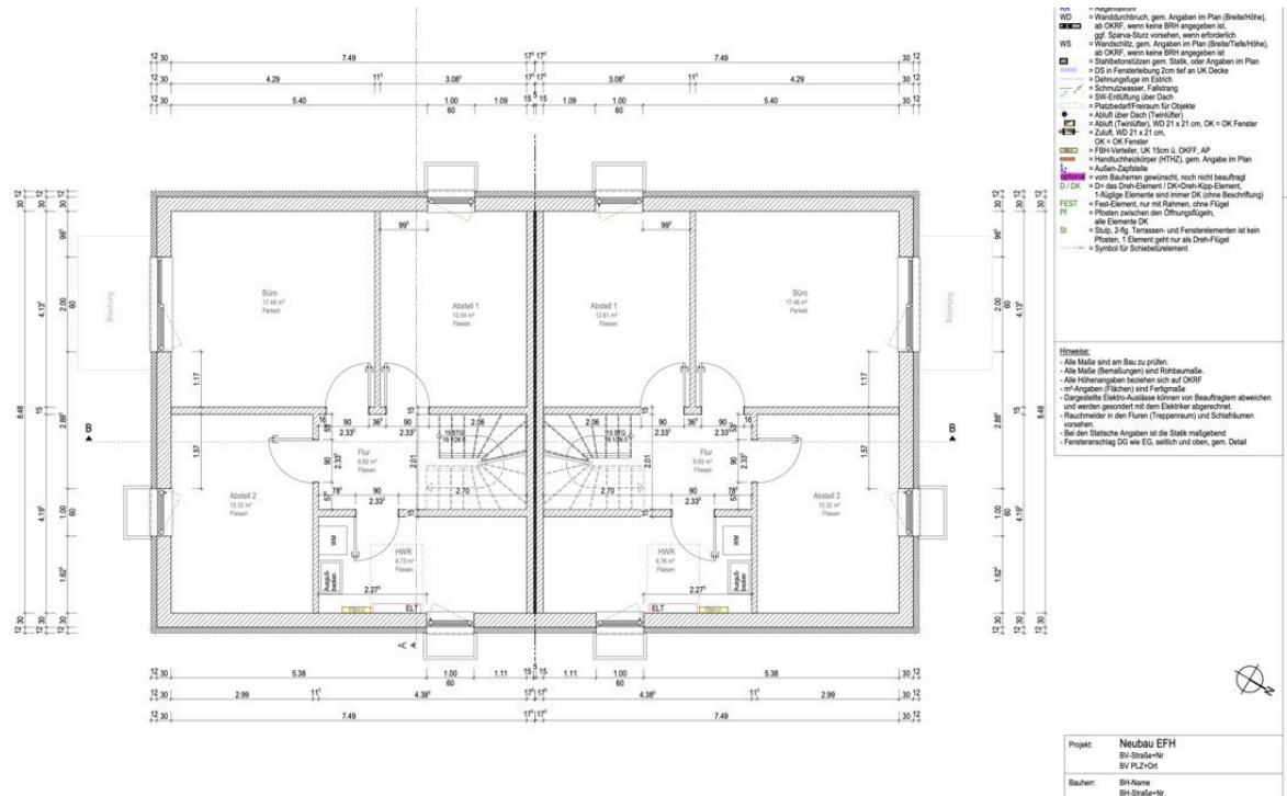
KG Grundriss DHH AB
