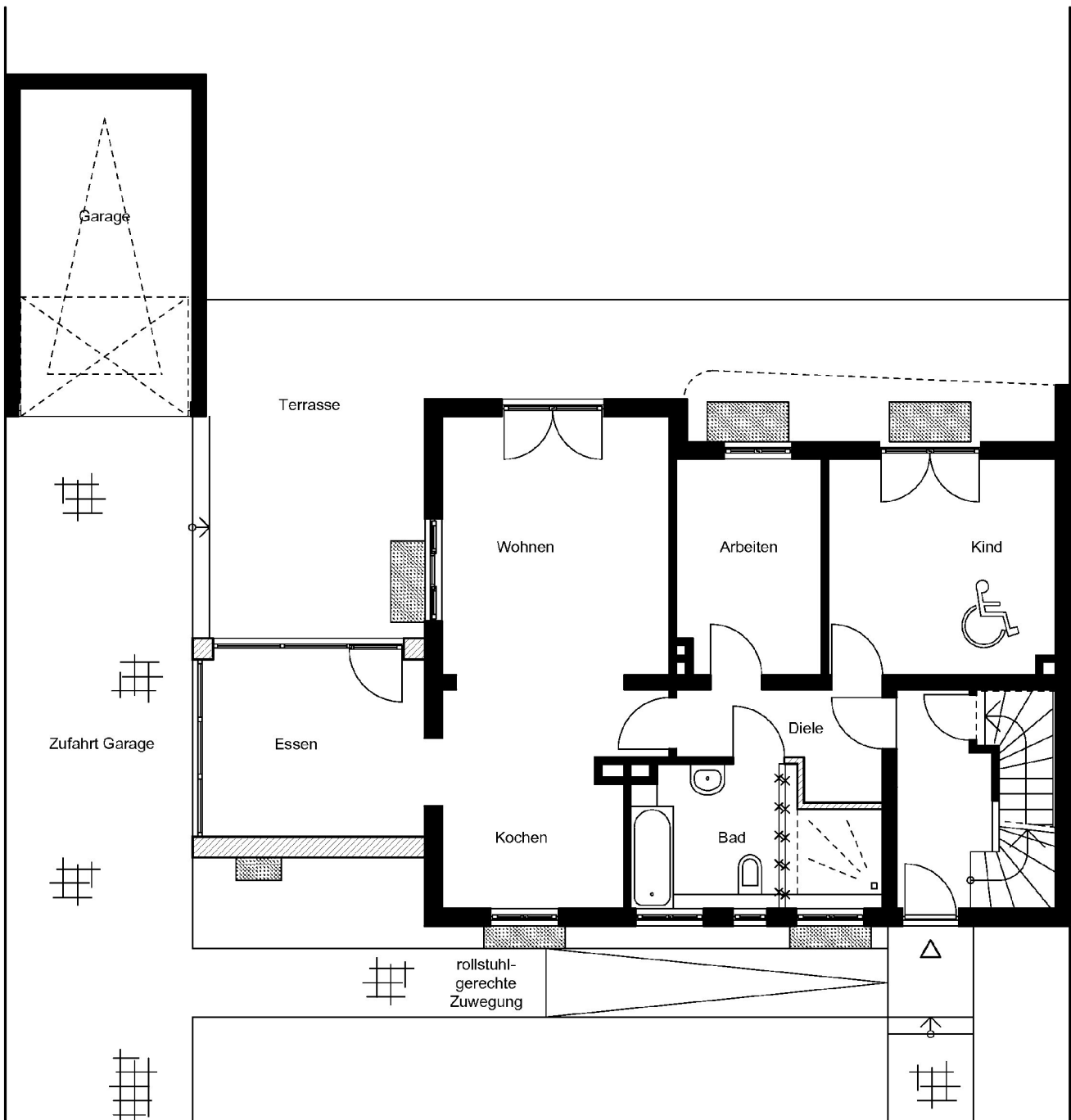
Abbildung 16: Grundriss Erdgeschoss
