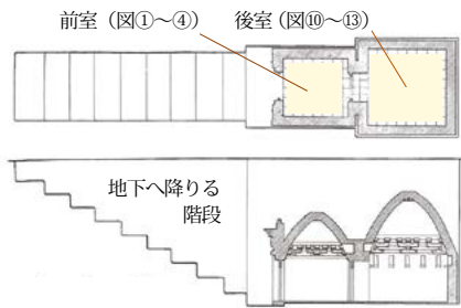
⑤ 墓の平面図と側面図
