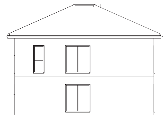
Ansicht Westen
