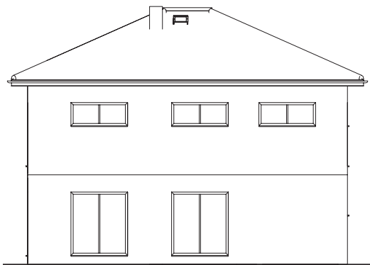
Ansicht Osten
