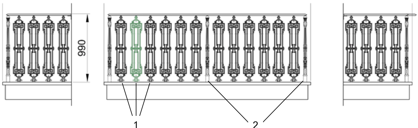
Horizontale Montage
