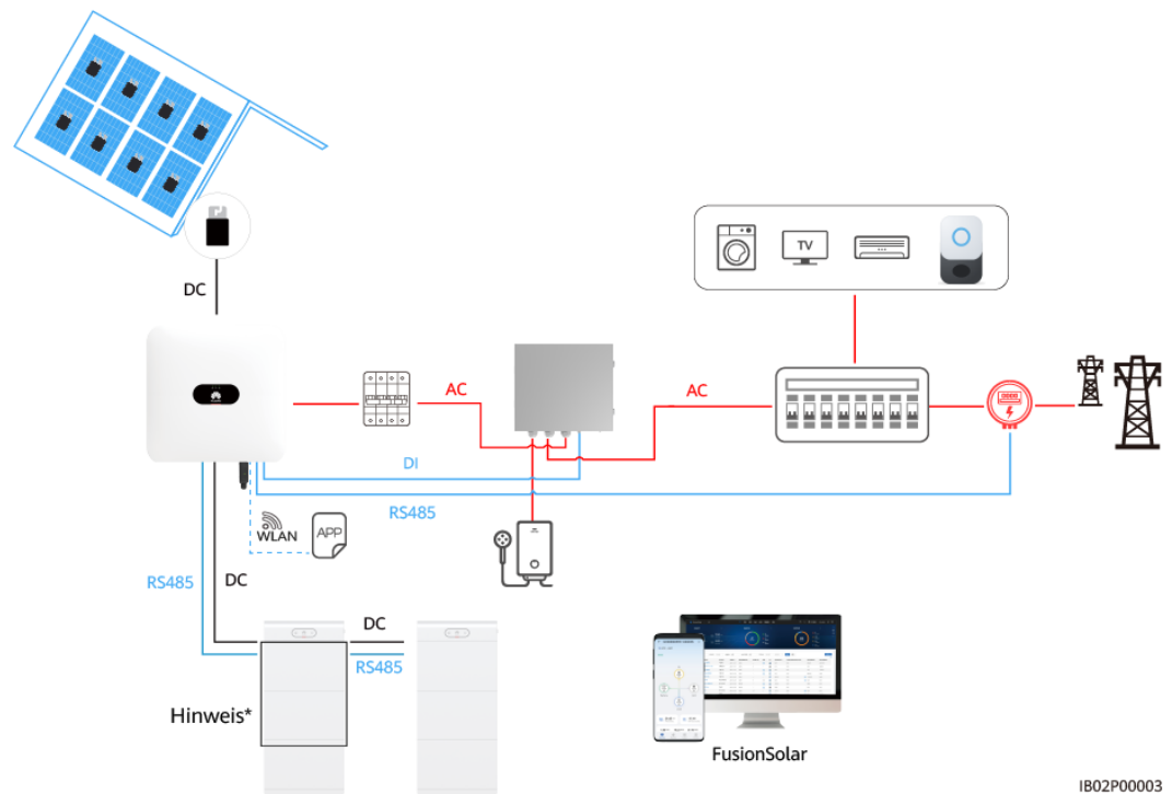
Abbildung 2-8 Netzgekoppeltes/-entkoppeltes Szenario
