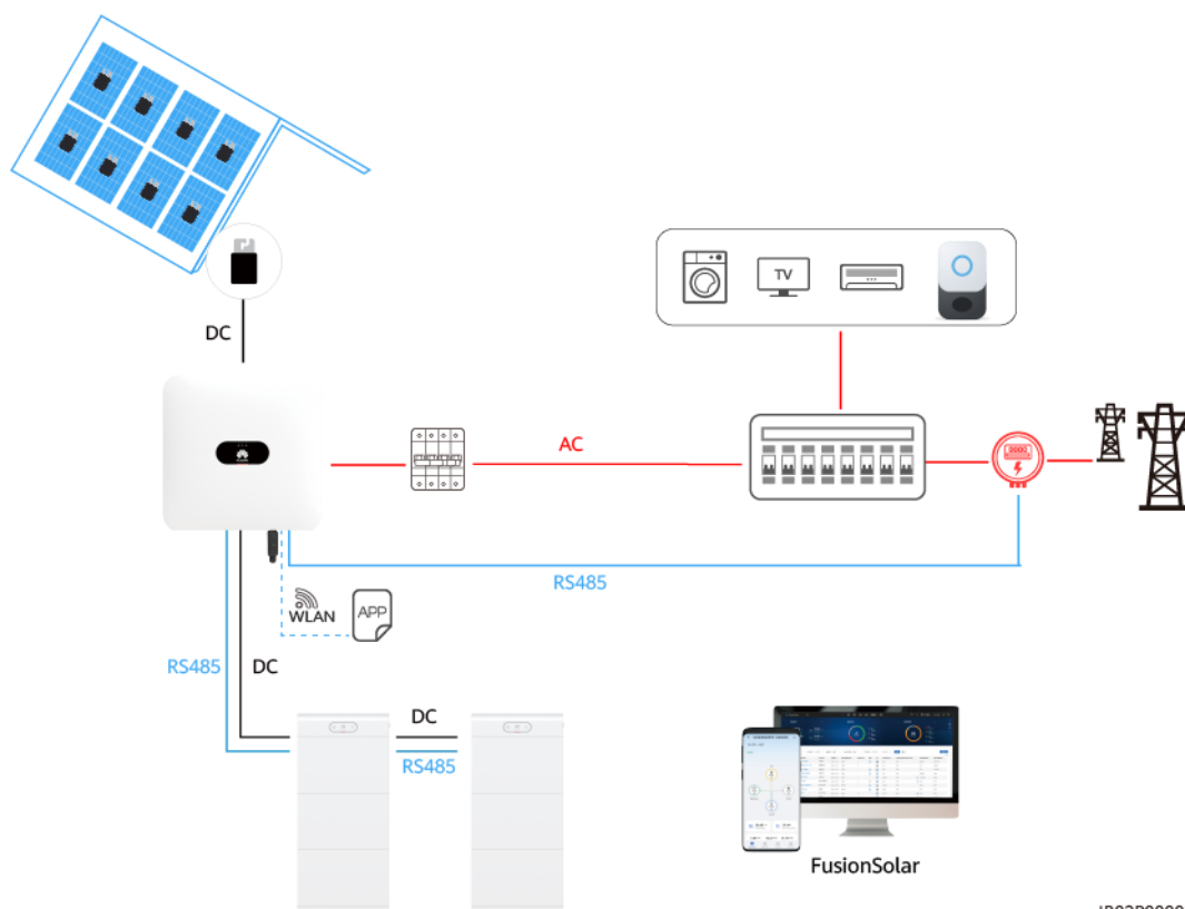
Abbildung 2-7 Netzgekoppeltes Szenario
