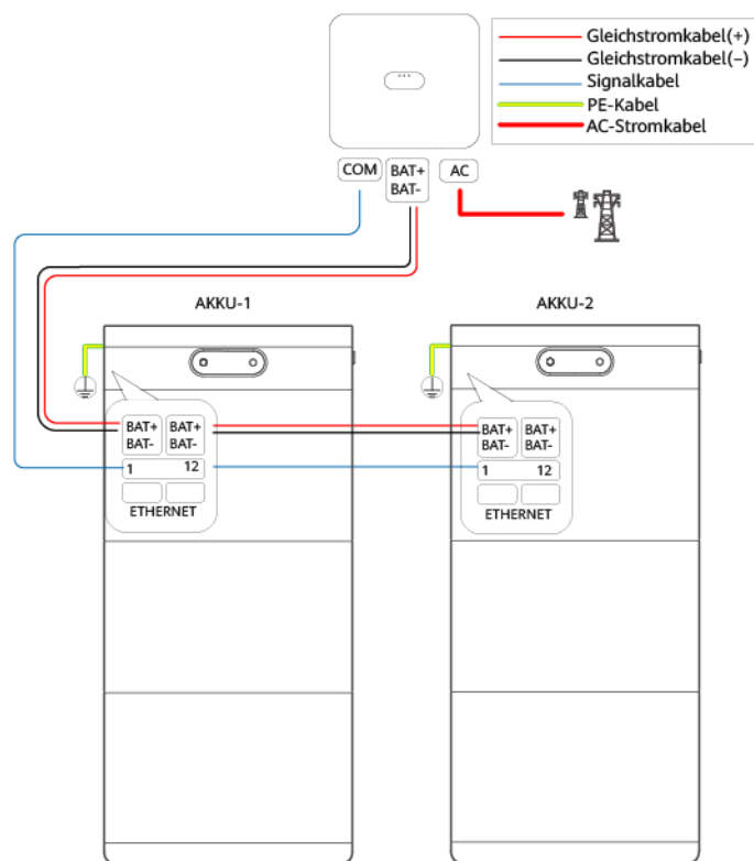
Abbildung 3-1 Kabelverbindungsplan
