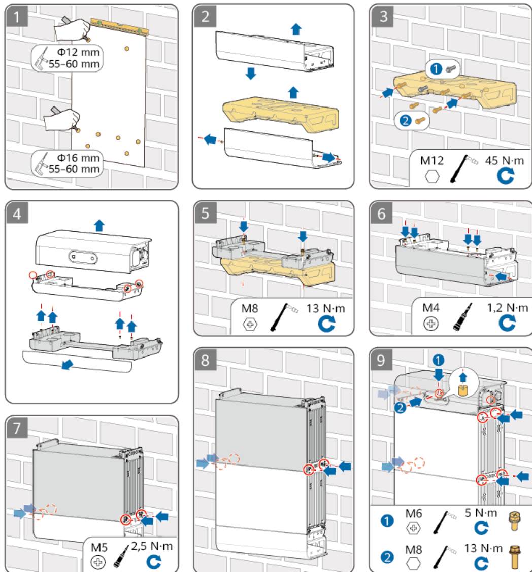
Abbildung 4-6 Wandmontage
