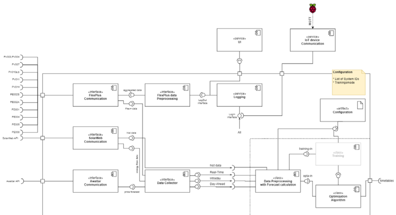
Abbildung 6: Softwarearchitektur Batteriepool
