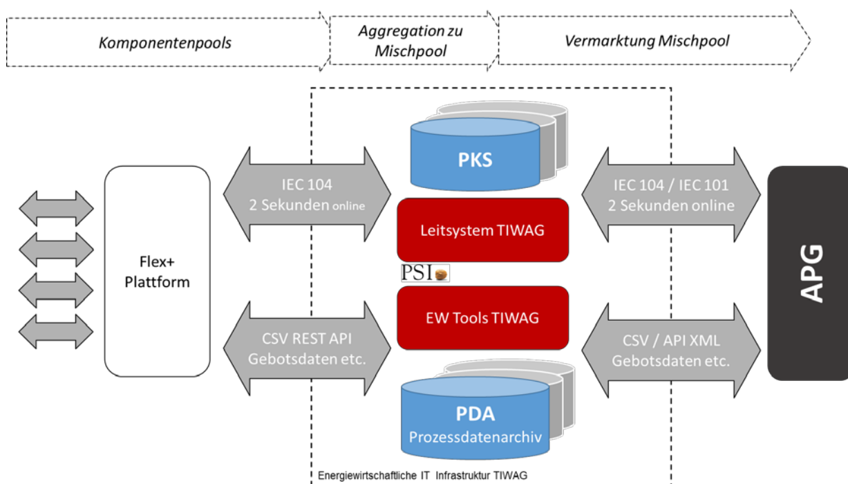
Abbildung 8: Softwarearchitektur Mischpool am Beispiel Regelreservevermarktung
