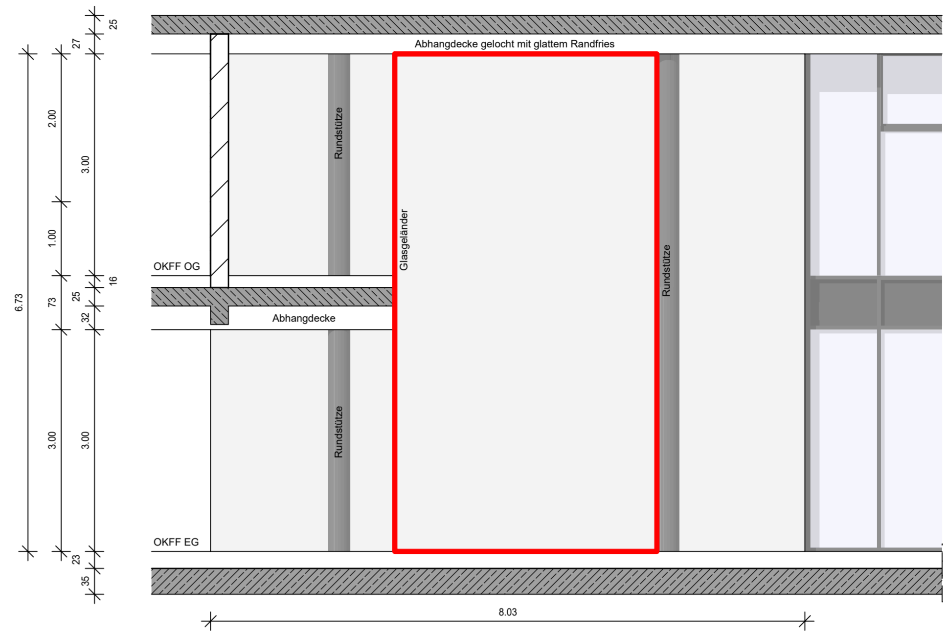
Ansicht Wandfläche
