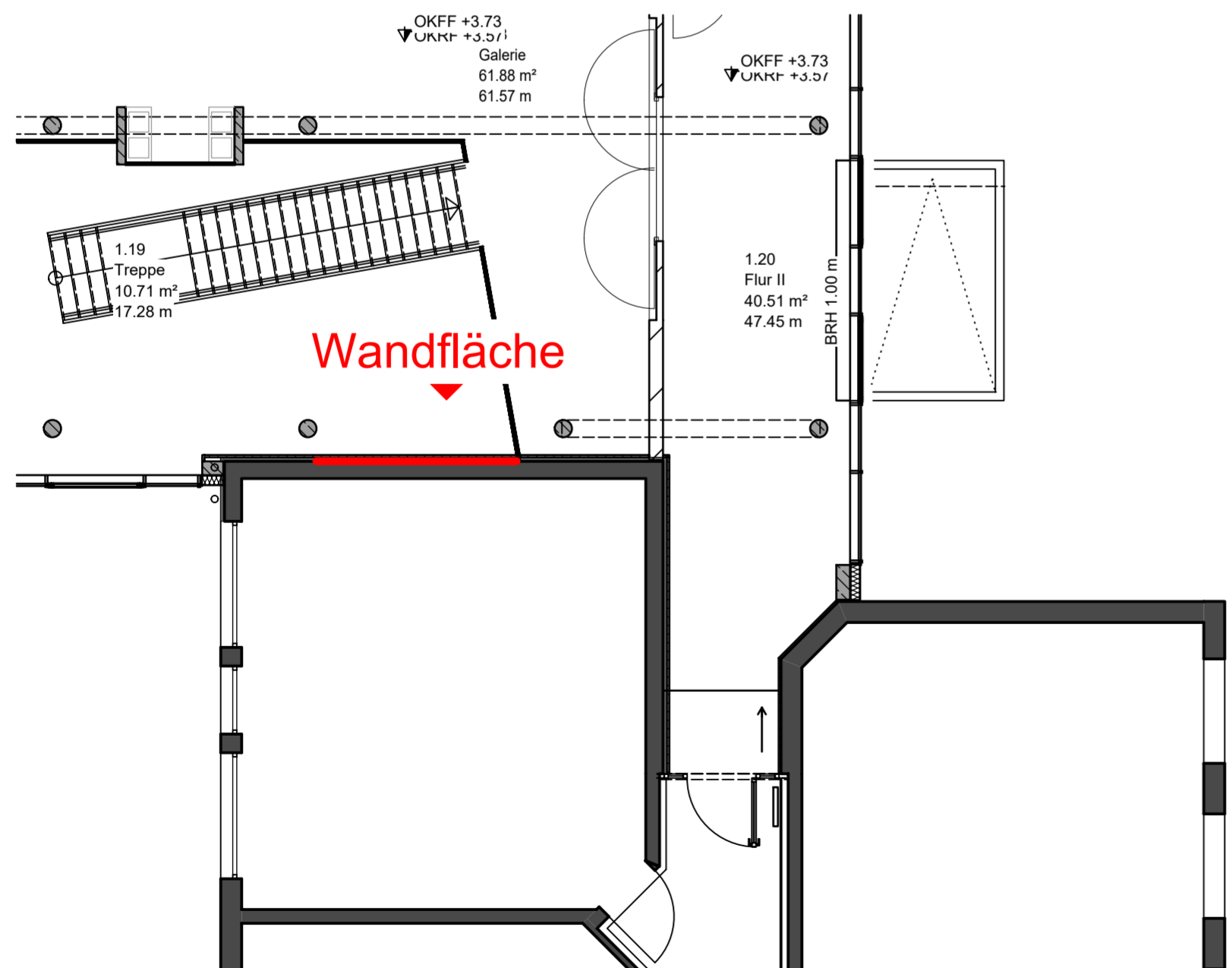
Ausschnitt Grundriss Obergeschoss
