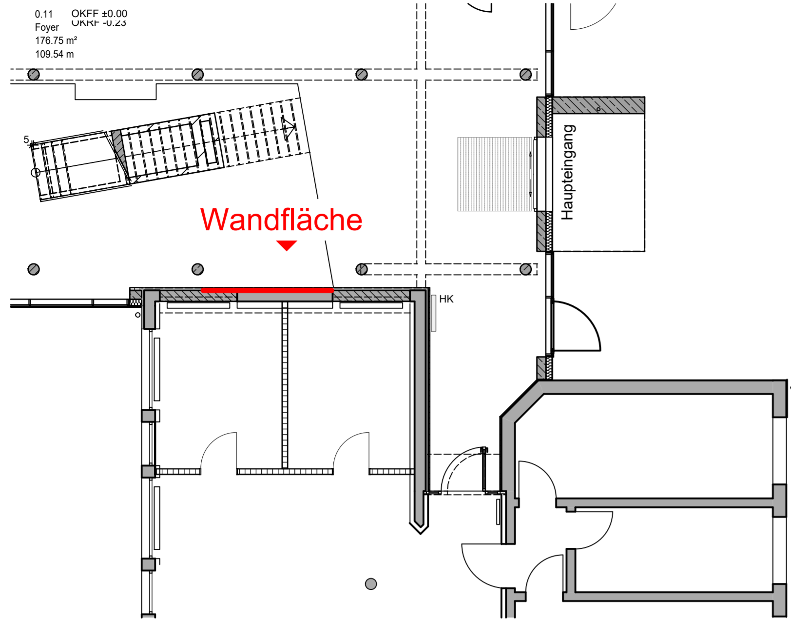
Ausschnitt Grundriss Erdgeschoss
