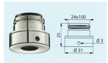
Anschluss M22 x 1 IG Antivandalismus- Ausführung AT821124
