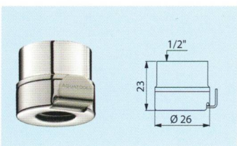
Anschluss G 1/2B AT820120
