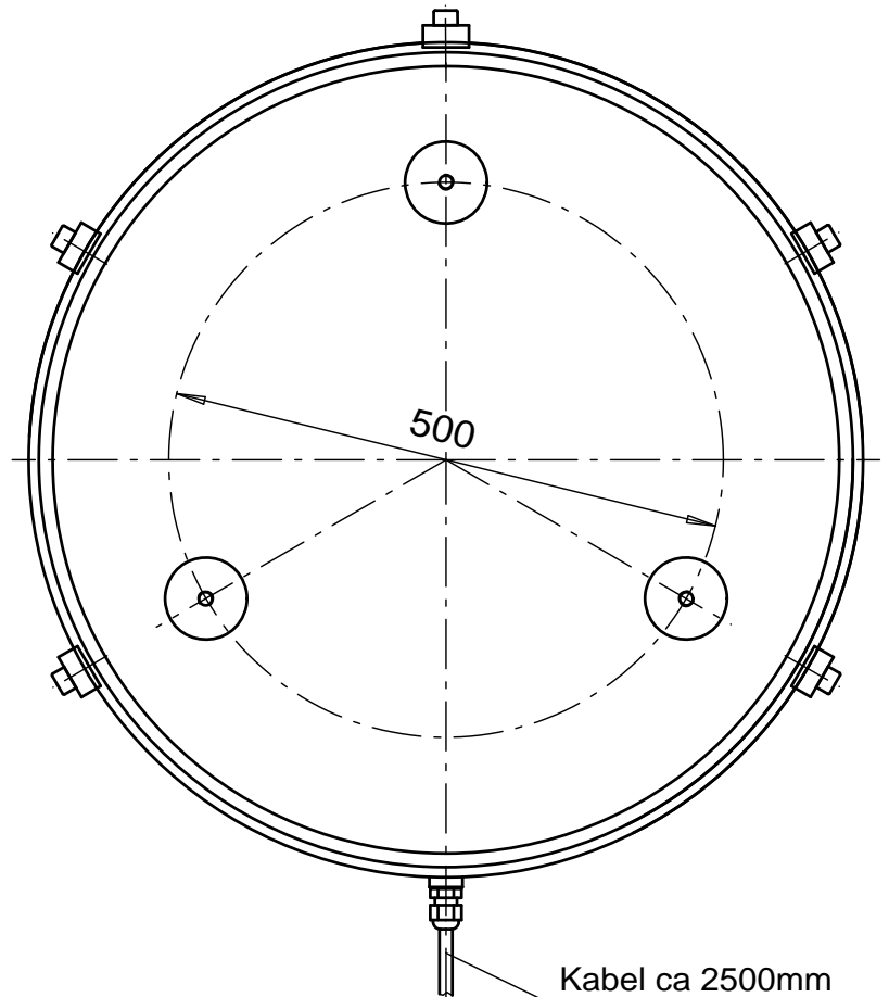
Ansicht von Unten
