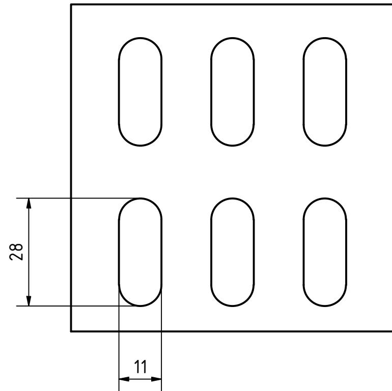
Lochbild ( 1 : 1 )
