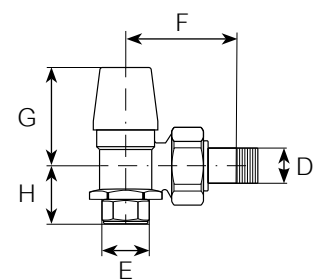
Eckventil
