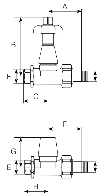
Durchgangsventil
