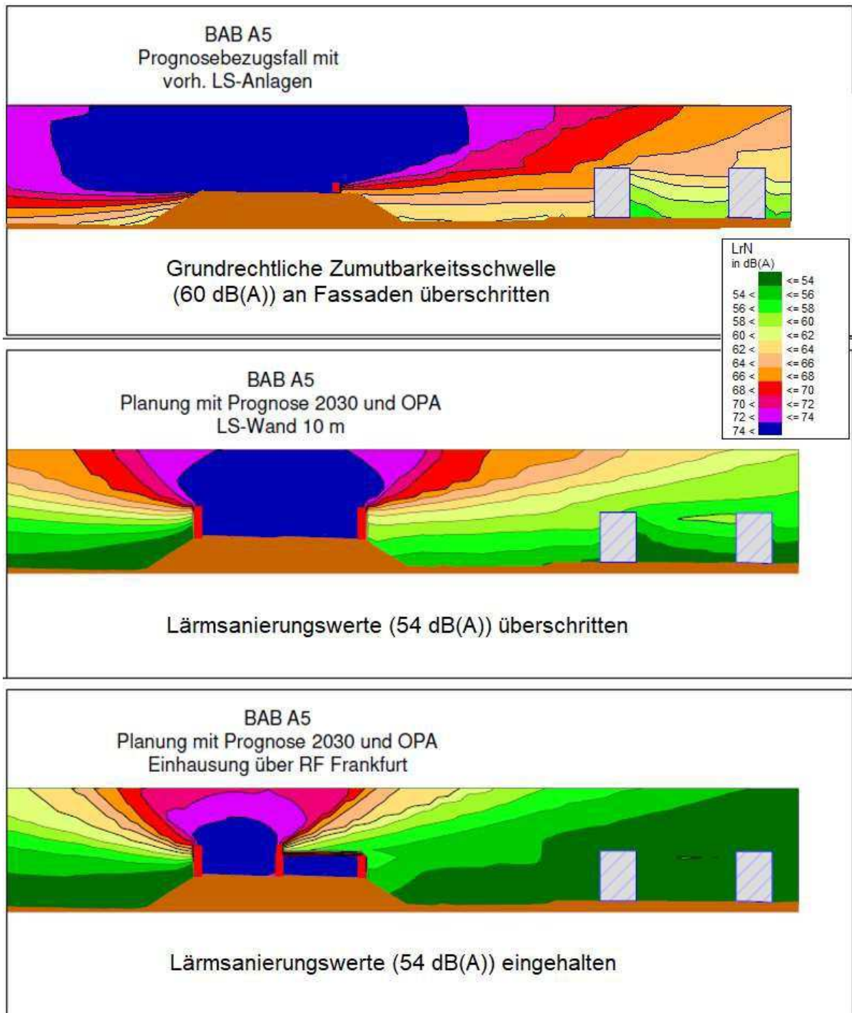
Abbildung 90: Schnittlärnkarte Schwarzerlenweg 52 - Nachtpegel
